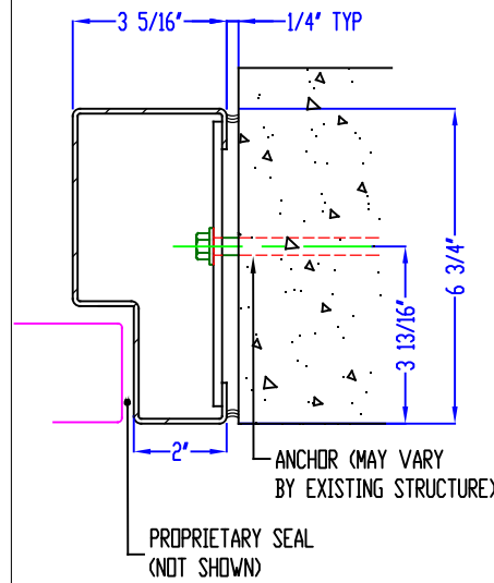
DETAIL C JAMB DETAIL ②④
